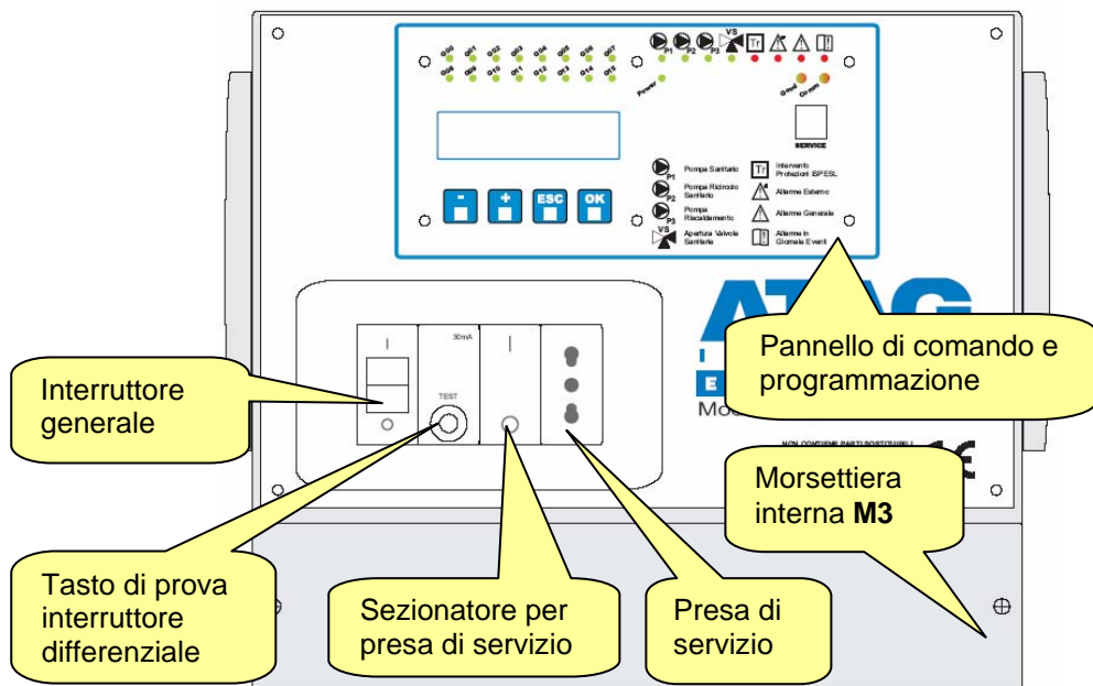
Fig. 4.1 – Quadro elettrico Supervisor
