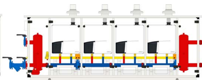
Fig. 2.4 – Modulo R+S speciale con equilibratore sanitario
