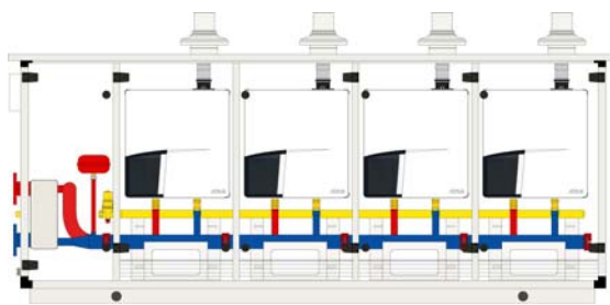
Fig. 2.3 – Modulo R speciale con scambiatore
