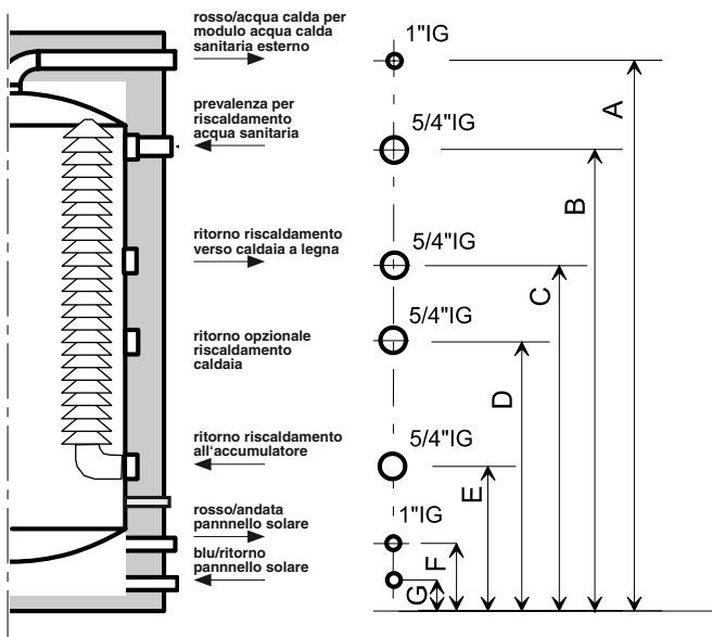
Misure degli allacciamenti all'accumulatore
