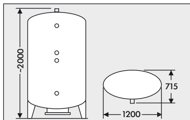
Imm. 19.1: Accumulatore Tampone Volume 1200 Litri Dimensioni in millimetri! Vedi anche "dati di misura" pagina 22
