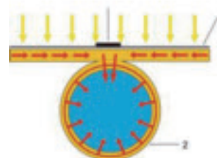
Rispetto alla precedente superficie assorbente (sotto), viene ora decisamente migliorata la conduzione del calore, grazie alla saldatura più ampia e alla minor distanza tra i tubi.
