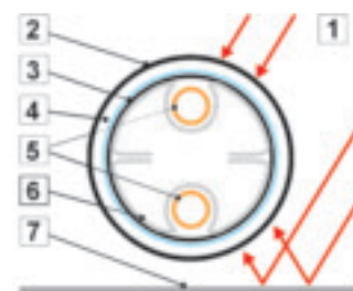
Principio dei tubi sottovuoto
